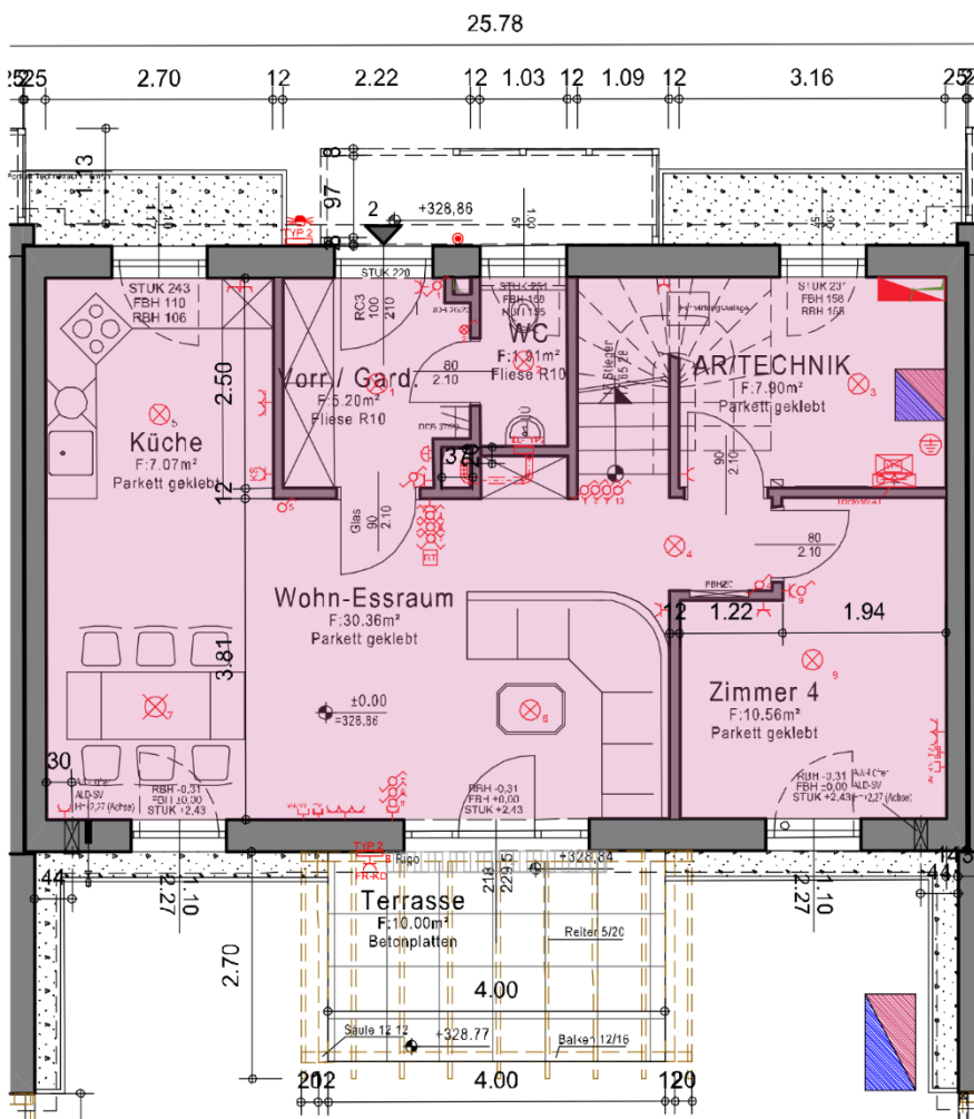
Erdgeschoss
