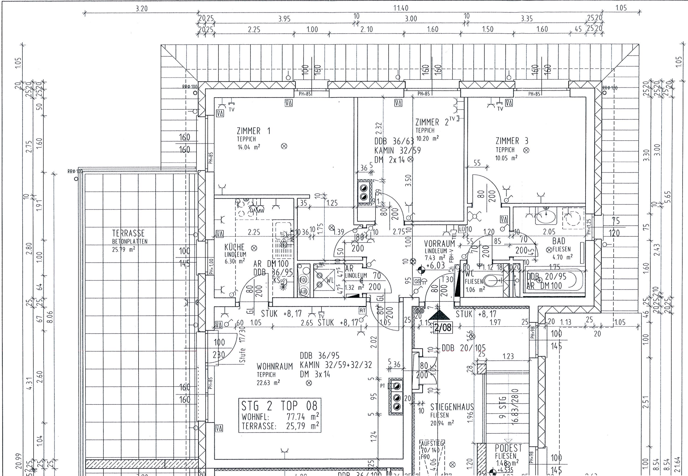
WHG HAUS2/20G/TOP8 M=1:50
