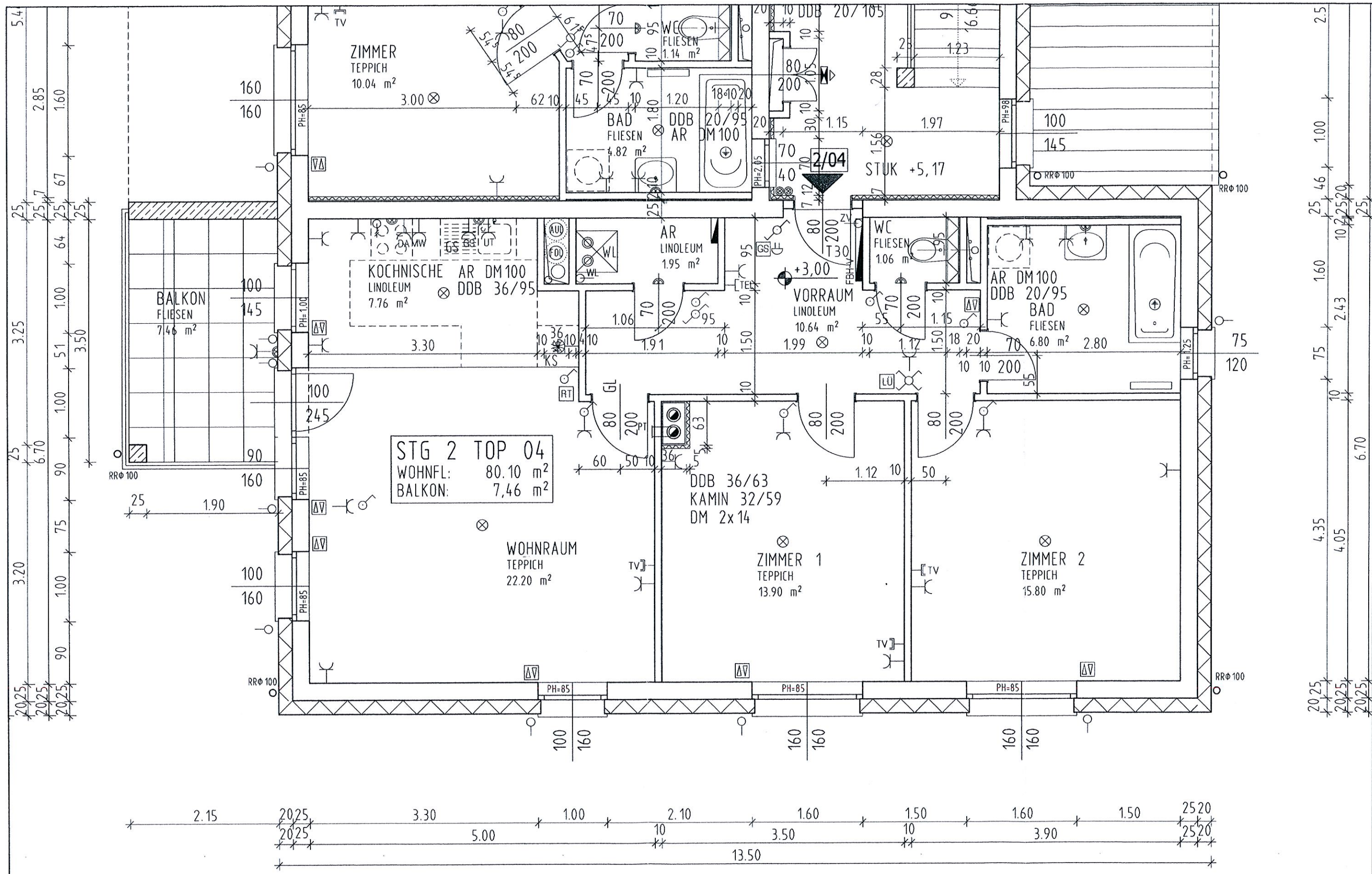
WHG HAUS2/10G/TOP4 M= 1:50
